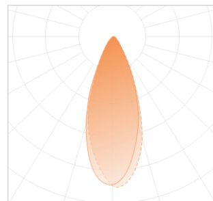
— C0-180 — C90-270 45°
